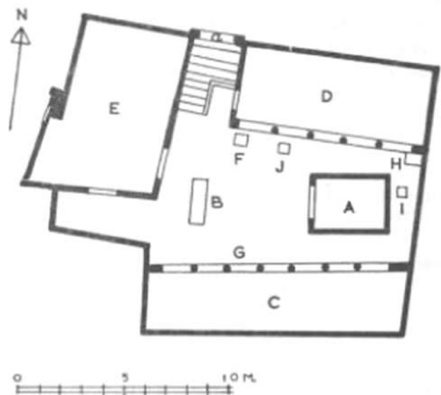
12. Κάτοψη του Σεραπειείου Α στη Δήλο. Το γράμμα «J» αντιστοιχεί στο κιβώτιο προσφορών του ναού.
