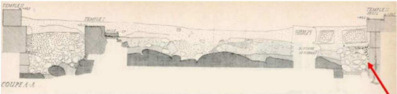
6. Στρωματογραφική τομή του ναού της Λητούς στην Ξάνθο και η θέση της προσφοράς θεμελίωσης.
